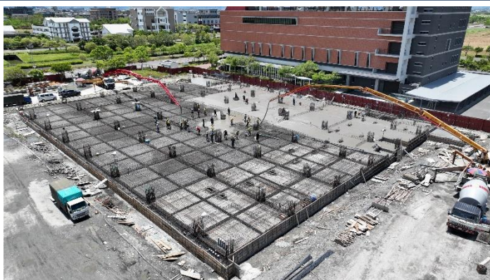
一樓板灌漿作業
