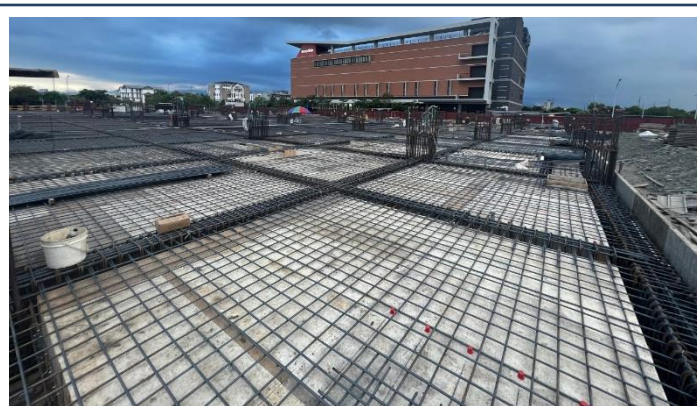
一樓版鋼筋綁紮
